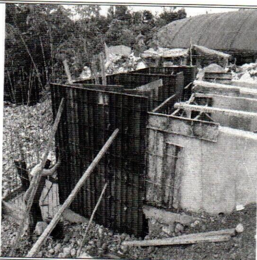
Foto No.5 Excacion y figuracion de hierro para el guaje del lavado de vehiculos.
