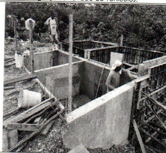
Foto No.6 Excacion y figuracion de hierro para el guaje del lavado de vehiculos.
